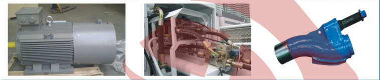
HBT series motor engine concrete pump HBT系列混凝土电机泵主要技术参数及配置
